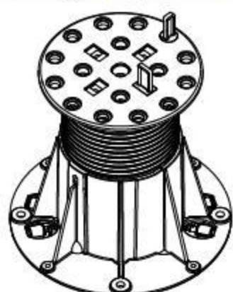
Regulowany wspornik BC-5 o zakresie od 100 do 200 mm
